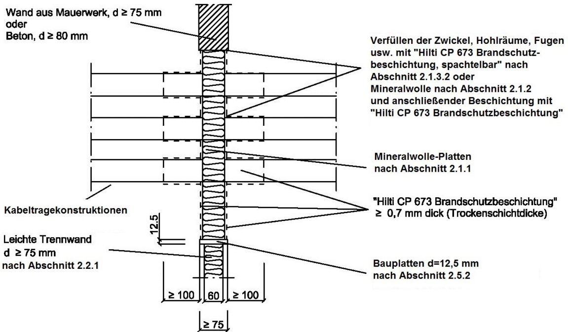
Schnitt A-A (Kabel nicht dargestellt)
