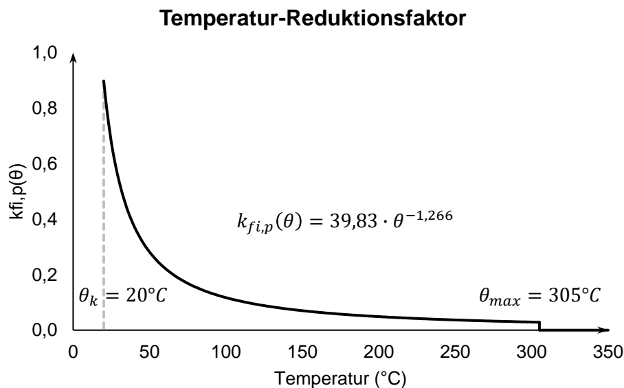
Abbildung C5: Reduktionsfaktor k_{fi,p}(\theta)
